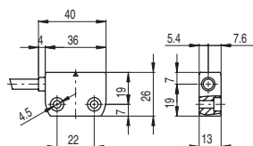
Sensore magnetico SR AL●●AN● con cavo integrato
