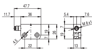
Sensore magnetico SR AL●●ALK con connettore M8
