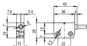
Sensore magnetico SR AL●●AN● con cavo integrato
