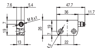
Sensore magnetico SR AL●●ALK con connettore M8
