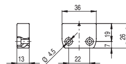
Azionatore codificato SM A01N
